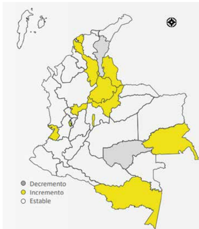
Figura 1: Comportamiento inusual de notificación de evento de interés: intento de suicidio en Colombia, periodo 2021-2022.
